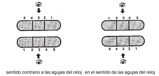
Elementos en apoyo lateral
